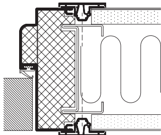
Vollspantür
