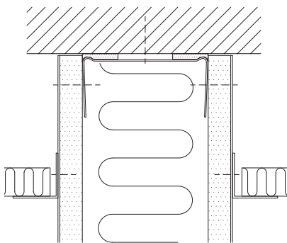
Abgehängter Deckenanschluss
