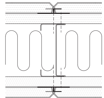
Gipsverbindung Typ 1290
