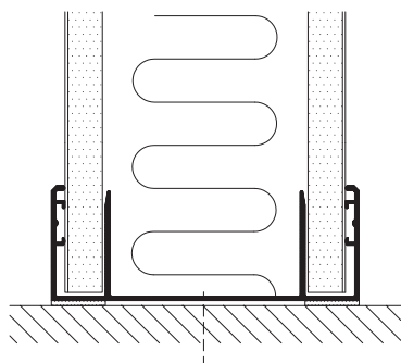
Bodenanschluss
