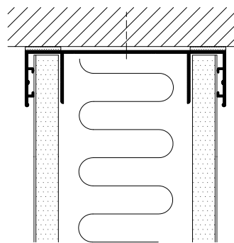
Fester Deckenanschluss
