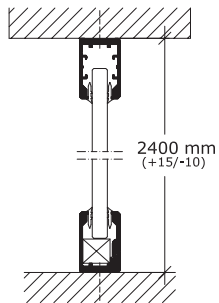
L1/L3 Senkrechter Schnitt
