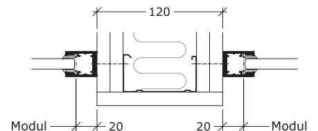
V7B Wandanschluss zwischen Querwänden
