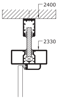
L4A-1 Aluminiumzarge mit 24 M Ganzglastür
