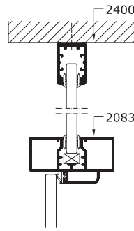
L4A-2 Aluminiumzarge mit 21 M Ganzglastür und oberer Verglasung
