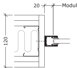
V7A Wandanschluss
