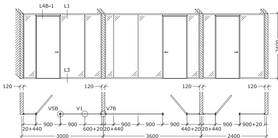
Beispiel 3: Grund- und Aufriss von DEKO FG Fast Verglasung zwischen Querwänden bei Gebäudemodul (beispielsweise 3000/3600/2400 mm)
