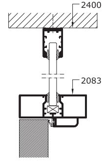
L4B-2 Aluminiumzarge mit 21 M Vollspantür und oberer Verglasung
