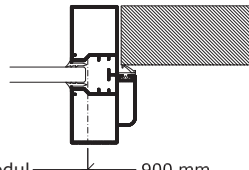
V5B Aluminiumzarge mit Vollspantür
