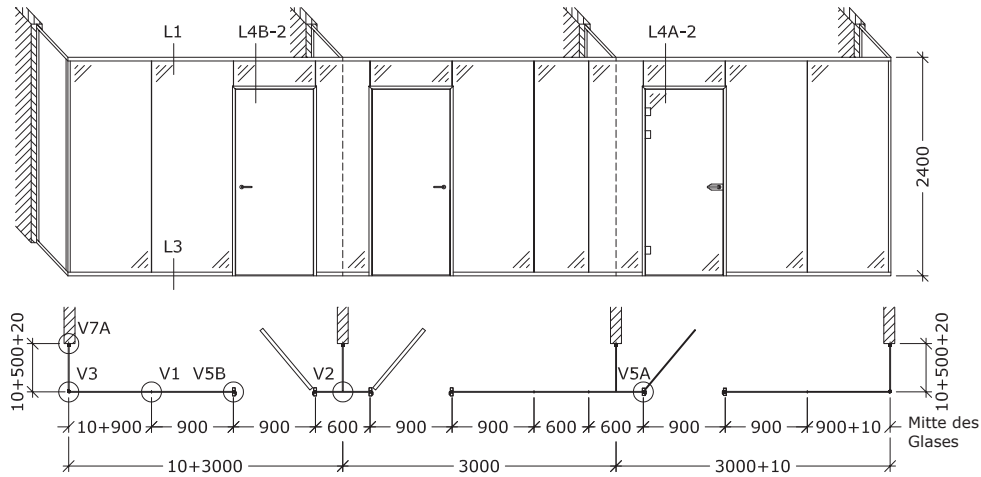
Beispiel 1: Grund- und Aufriss von DEKO FG Fast bei Gebäudemodul 3000 mm
