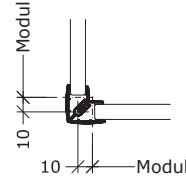
V3 90° Ecke
