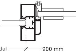
V5A Aluminiumzarge mit Ganzglastür
