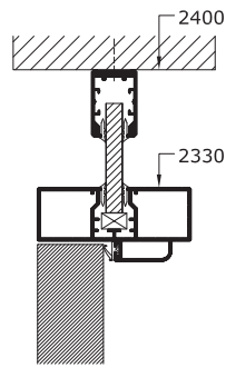
L4B-1 Aluminiumzarge mit 24 M Vollspantür
