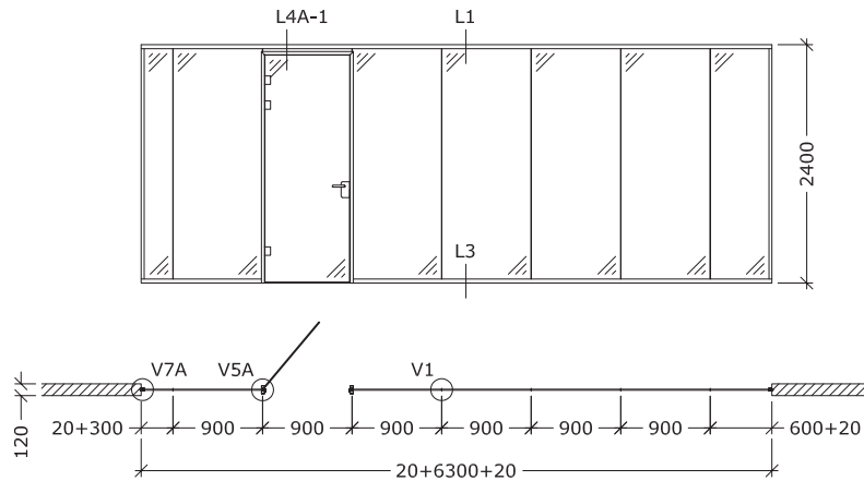
Beispiel 2: Grund- und Aufriss von DEKO FG Fast in beliebiger Wandöffnung
