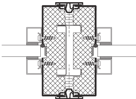
Glasverbindung - Einzelverglasung
