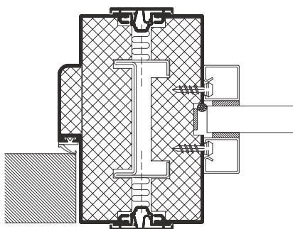
Tür-Glasverbindung
