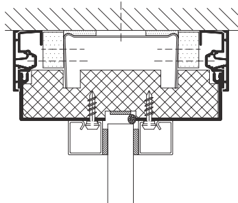
Deckenanschluss
