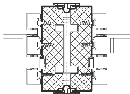
Glasverbindung – Doppelverglasung mit Jalousien
